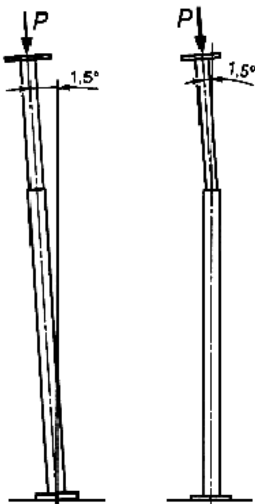
Рисунок 14 - Схема испытания составных стоек
