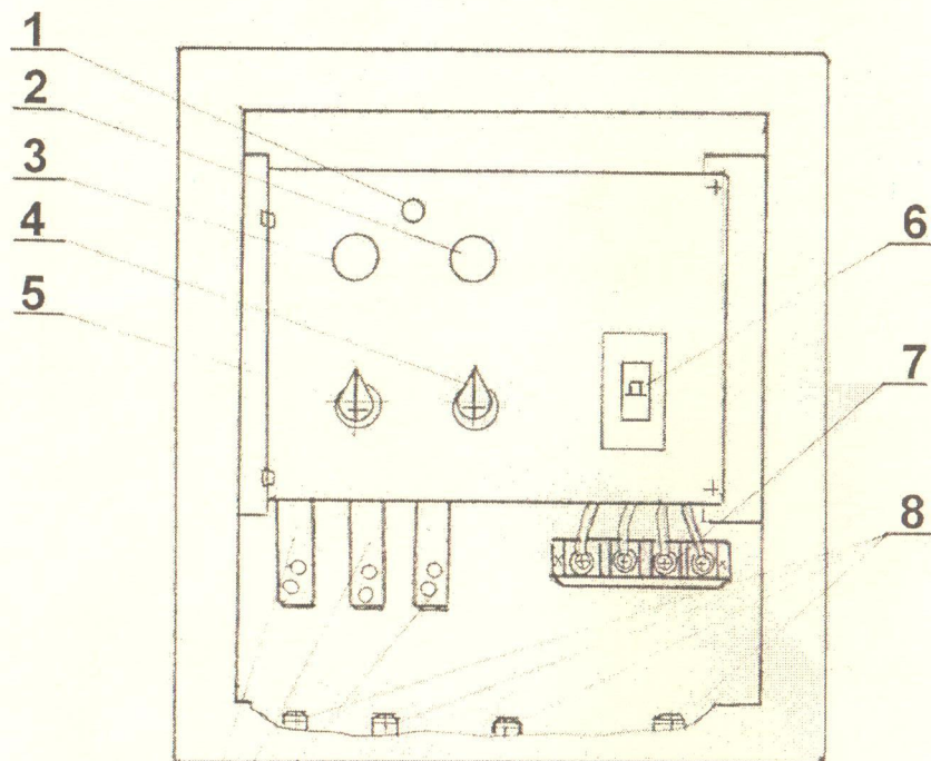
Шкаф управления (вид при снятой двери)
