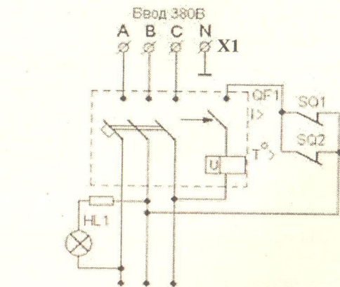
Схема электрическая принципиальная КТПТО - 80
