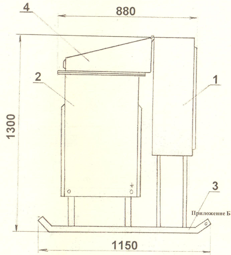
Рис.1 Комплексная трансформаторная подстанция КТПТО-80-У1
